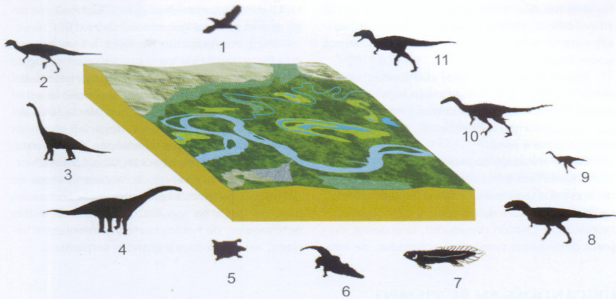
Figura 4. Reconstrucción paleoambiental de la Formación Portezuelo, mostrando importante vegetación herbácea con ríos meandrosos y lagunas abandonadas. Los principales vertebrados terrestres de esta unidad corresponden a los siguientes taxones (no a escala): 1) ave neornite, 2) iguanodonte mediano, 3) titanosaurio basal, 4) titanosaurio avanzado grande, 5) tortugas quéelidas y podocnemoideas (de agua dulce), 6) cocodrilo notosuquio, 7) pez pulmonado ceratodontiforme, 8) carcarodontosáurido, 9) alvarezsáurido, 10) dromeosáurido unenlagino y 11) abelisáurido.
