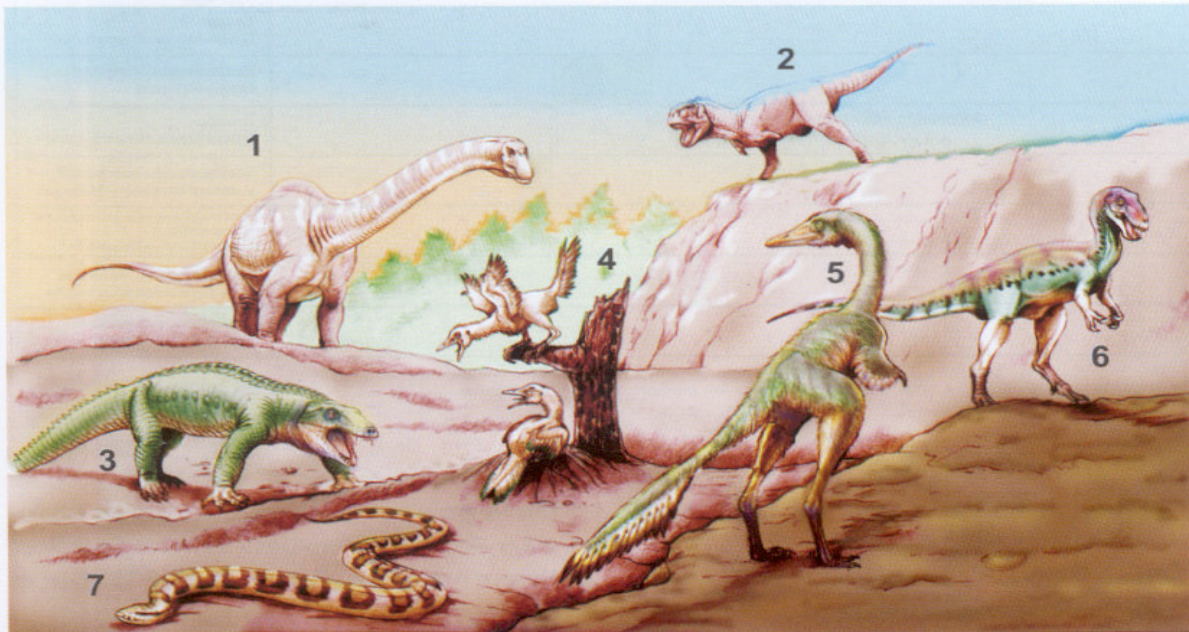
Figura 5. Reconstrucción de la fauna de tetrápodos del Subgrupo Río Colorado, según una ilustración preparada por Jorge González. 1) titanosaurio, 2) abelisáurido, 3) cocodrilo notosuquio, 4) ave enantiornite, 5) alvarezsáurido, 6) abelisáurido noasaurino y 7) serpiente dinilísida.
