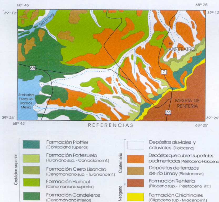
Figura 2. Bosquejo geológico de la comarca de El Anfiteatro, basado en Hugo y Leanza (2001a).
