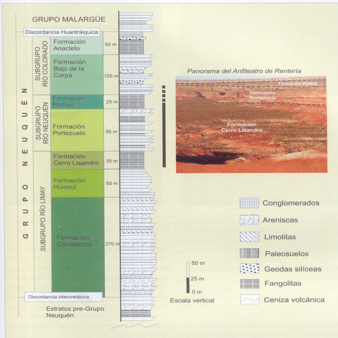
Figura 3. Columna estratigráfica idealizada del Grupo Neuquén, basado en Leanza (1999). La barra vertical negra indica el tramo estratigráfico que es posible observar en El Anfiteatro y, en guiones, el tramo basal de la Formación Bajo de la Carpa, bien expuesta 10 kilómetros al nordeste de esta localidad.
