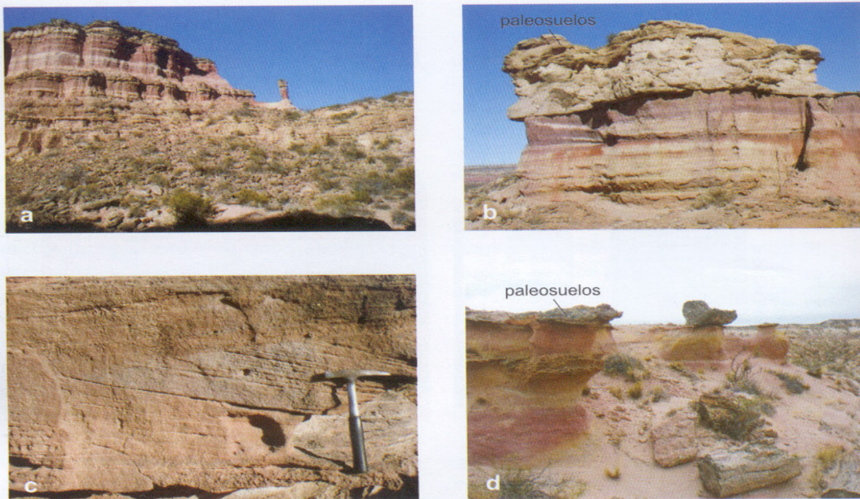
Fotografía 3. Aspecto general de la Formación Portezuelo: a) algunas estructuras relicticas labradas por la erosión; b) niveles arenosos cubiertos por paleosuelos; c) detalle de estratificación cruzada indicativa de ríos meandrosos; d) aspecto de paleosuelos con preservación de troncos de árboles silicificados de mediano porte.
