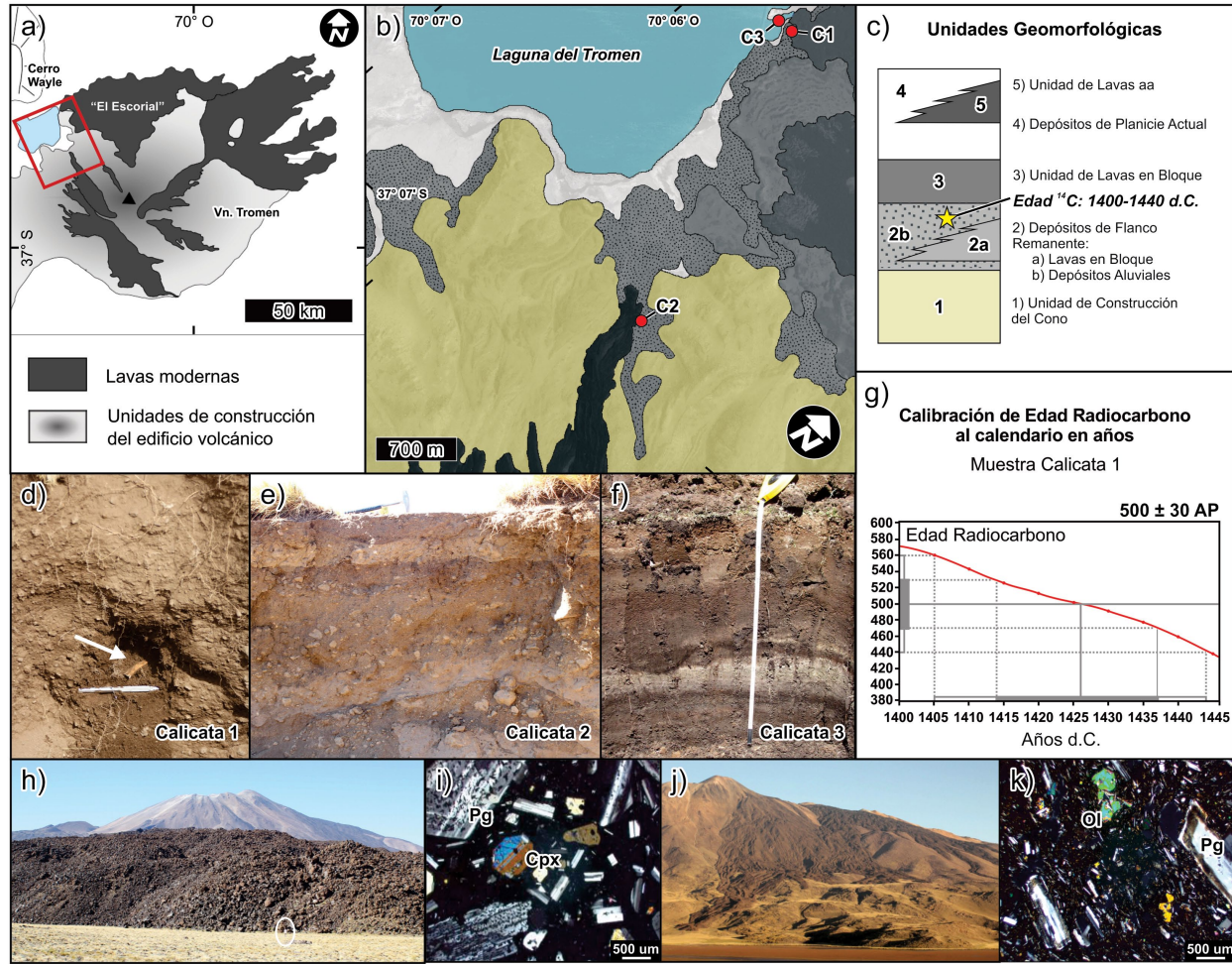
Figura 1: a) Figura esquemática del volcán Tromen (en el recuadro se detalla el área de estudio). b) Mapa geomorfológico del sector NO del volcán Tromen. (C1= Calicata 1, C2 Calicata 2, C3 = Calicata 3). c) Columna estratigráfica esquemática mostrando la relación de las unidades geomorfológicas presentes. d) Calicata 1. Detalle de los Depósitos de Aluviales Remanentes en facies distales (La flecha muestra localización del fósil de vertebrado recolectado para el análisis radiocarbono). e) Calicata 2. Detalle de las facies aluviales remanentes en sectores proximales. f) Calicata 3. Facies lacustres de la Unidad de Planicie Actual. Se muestran los depósitos masivos de arenas finas limosas y minoritariamente a arcillas. g) Diagrama de edad radiocarbono convencional (método AMD - Beta Analytic Radiocarbon Dating Laboratory). Resultado calibrado 2\sigma : 1400 - 1440 d.C. 95 % de probabilidad. h) Unidad de Lavas en Bloque. Lóbulo frontal de la colada El Escorial (Persona de escala marcada con un círculo). i) Microfotografía de la colada El Escorial (Pg=Plagioclasa, Cpx = Clinopiroxeno). j) Vista general de la Unidad de Lavas aa. k) Microfotografía de la facies de lavas de la Unidad de Lavas aa (Pg = Plagioclasa, Ol = Olivina).
