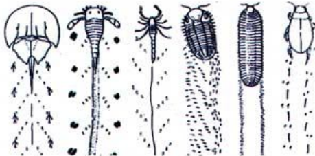
Figura 6. Algunos ejemplos de «trazas fósiles» formadas por el desplazamiento de organismos invertebrados en el fondo marino.
