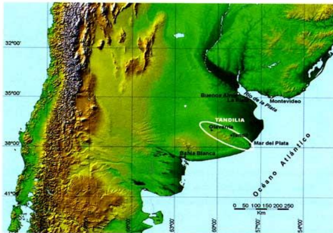
Figura 1. Ubicación regional del cordón de Tandilia.
