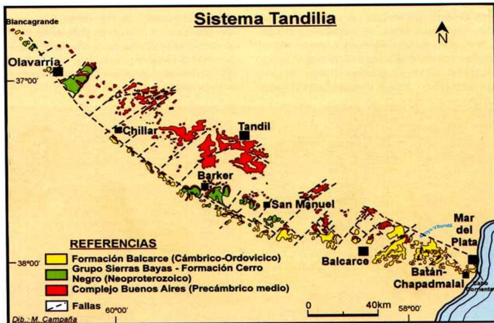
Figura 3. Bosquejo geológico general de Tandilia.
