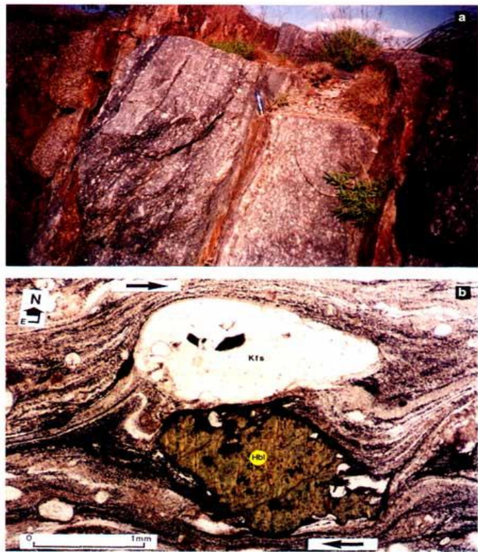
Fotografía 2. a) Rocas deformadas del Complejo Buenos Aires en Boca de la Sierra. b) Fotografía del corte microscópico de una roca; las estructuras originadas por la deformación permiten interpretar la dirección y sentido de los esfuerzos, indicados por las flechas.
