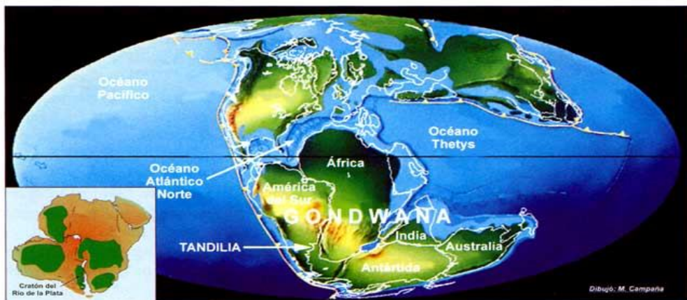
Figura 5. El supercontinente de Gondwana y la posición de Tandilia. Ésta forma parte de un núcleo continental antiguo llamado Cratón del Río de la Plata.
