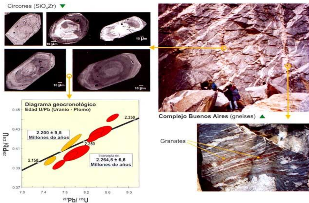
Figura 4. Afloramientos de rocas metamórficas (gneises ricos en granates) del Complejo Buenos Aires en la zona de Balcarce. Se muestran también cristales de circon obtenidos de estas rocas, cuya edad es de aproximadamente 2.200 millones de años, según el diagrama geocronológico.
