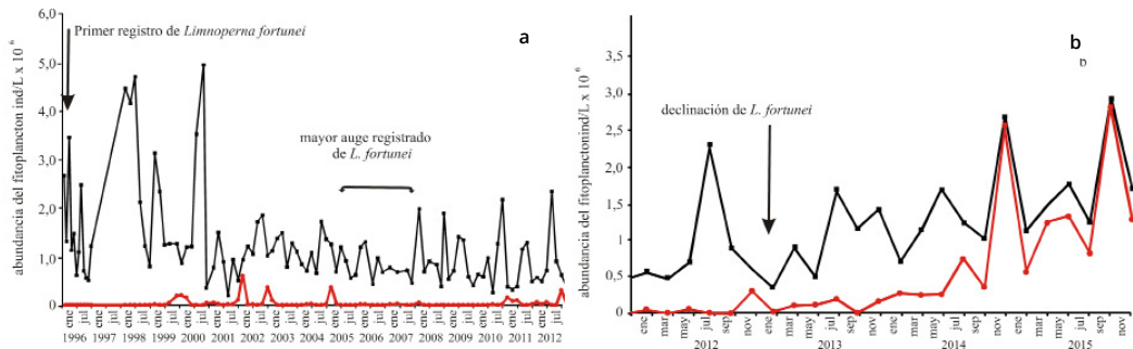
Figura 4. Variación temporal de la abundancia de algas fitoplanctónicas (línea negra) y de Ceratium hirundinella (línea roja) en la zona fótica de la estación Garganta: a) entre 1996 y 2012; b) entre 2012 y 2015.
